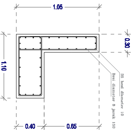
Balok Tumpu 1 : 25
