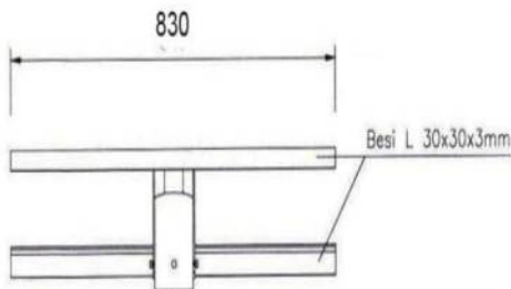
TAMPAK BELAKANG
