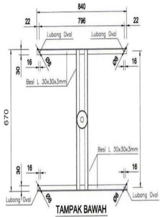
PENYANGGA PV MODULES 1 x pv 90 Wp
