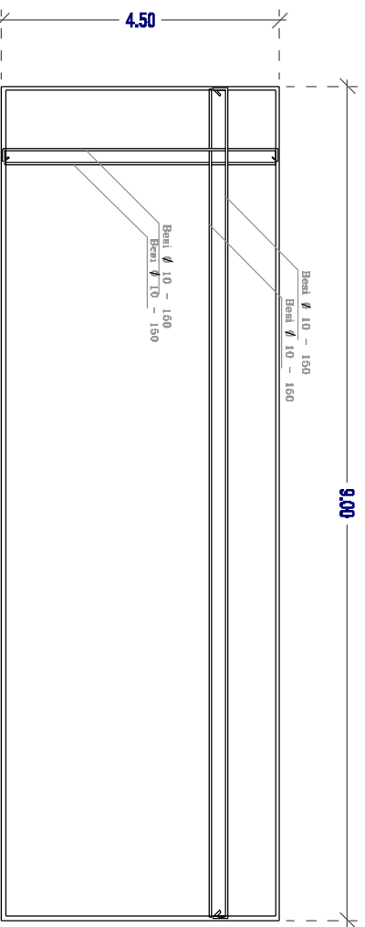
Penulangan Plat lantai 1 : 100
