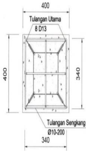
TAMPAK ATAS
