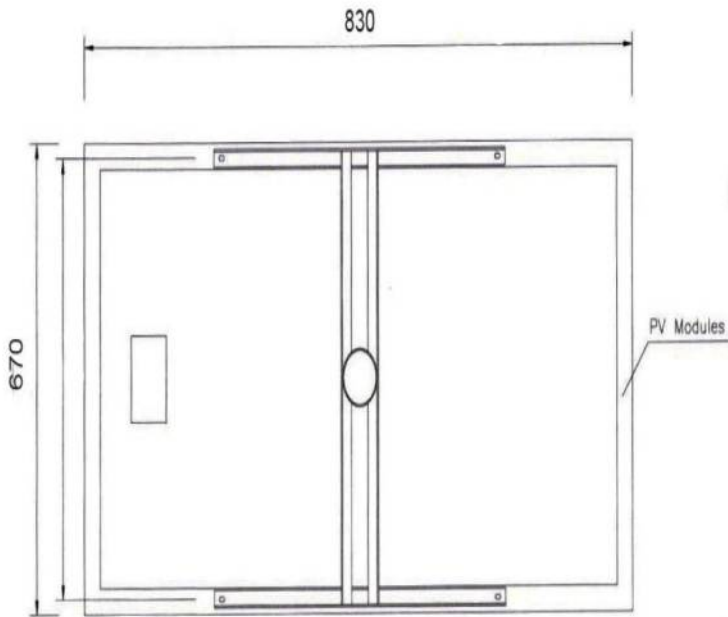
PENYANGGA PV MODULES 1 x pv 90 Wp
